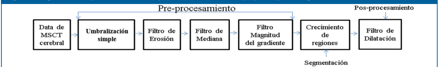
Figura 3. Diagrama de bloques de la técnica computacional no lineal (NLCT) propuesta para la segmentación del IVH
